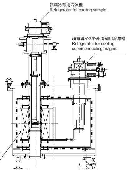
超電導マグネット Superconducting magnet
