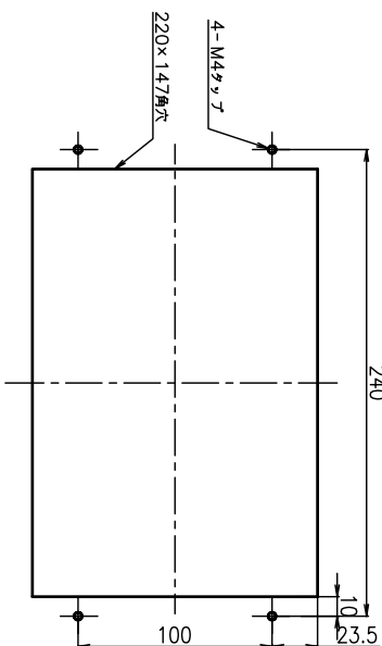
Z軸詳細(2:1)
